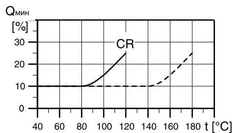
Рис. 28 Минимальная подача
