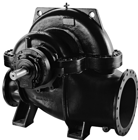
Рис. 1 Насос Grundfos LS
