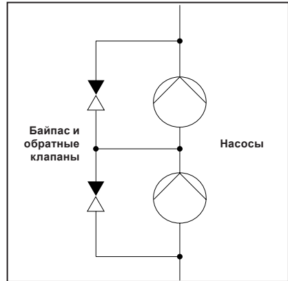
Рис. 14 Последовательно включенные насосы
