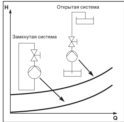
Рис. 12 Характеристики трубопровода
