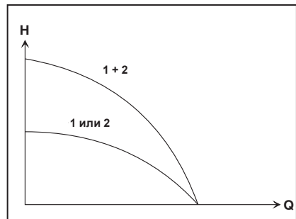
Рис. 15 Два однотипных насоса, включенных последовательно
