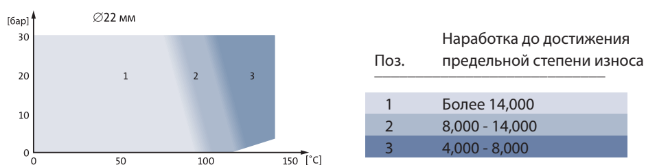
Рис. 3.12. График давления/температуры, отражающий срок службы уплотнения вала типа H из графита/SiC в воде для вала диаметром 22
