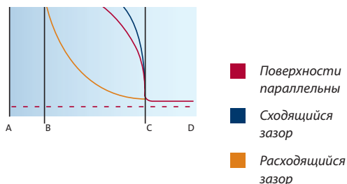
Рис. 1.22: Распределение гидростатического и гидродинамического давлений для различных геометрий зазора уплотнения
