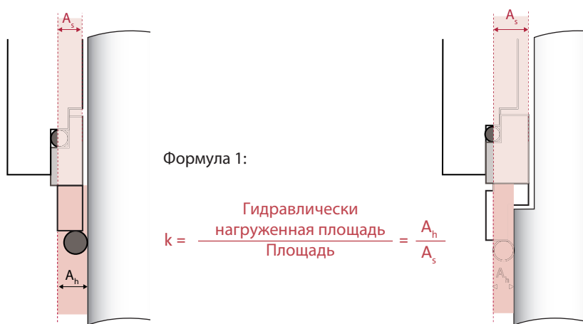
Рис. 1.15b: Сбалансированное уплотнение вала, k < 1
