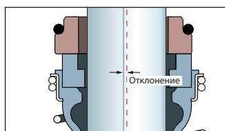
Рис. 5.15. Уплотнение вала с радиальным отклонением
