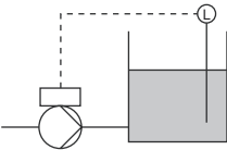
Fig. 37 "Konstant niveau"
