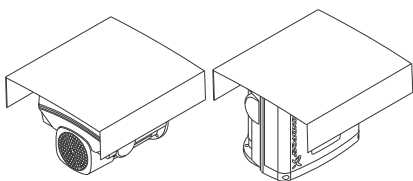
Fig. 2 Eksempler på overdækninger, leveres ikke af Grundfos
