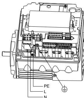
Fig. 5 Nettilslutning, 1-fasede motorer
