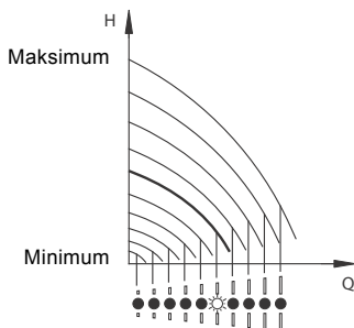
Fig. 17 Pumpe i reguleringsformen konstantkurve
