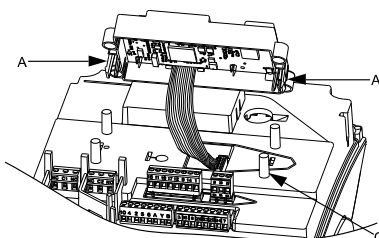
Fig. 68 Sådan placeres plastdækslet
