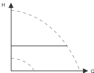
Fig. 30 "Konstant differenstryk"
