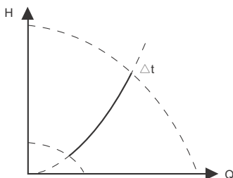
Fig. 32 "Konstant differensstemperatur"
