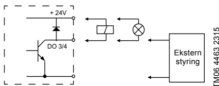
Fig. 42 Eksempel på konfigurerbare digitale indgange eller udgange
