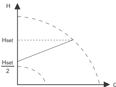
Fig. 24 "Proportionaltryk"
