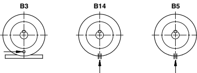
Fig. 3 Drænhuller
