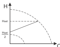
Proportionaltryk
