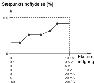
Fig. 49 Indflydelsestabel, eksempel med fem punkter
