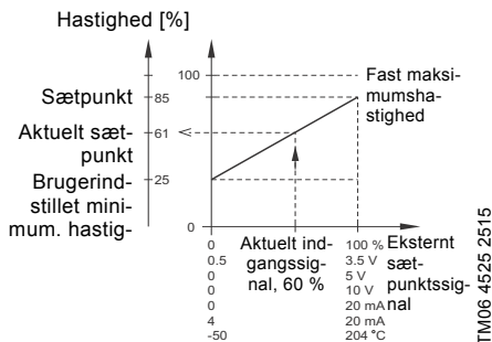
Fig. 46 Eksempel på sætpunktsindflydelse med konstantkurve
