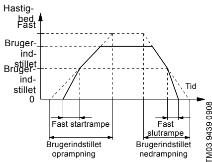
Fig. 52 Oprampning og nedrampning
