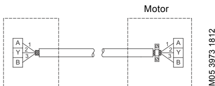
Fig. 10 Tilslutning med skærmet 3-lederkabel
