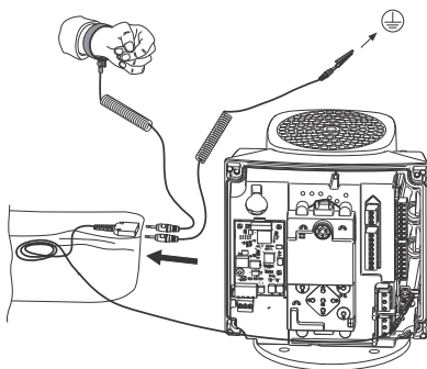
Fig. 54 Antistatisk servicesæt
