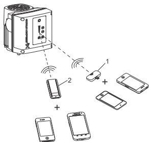
Fig. 22 Grundfos GO kommunikerer med pumpen via radiokommunikation eller infrarød forbindelse, IR
