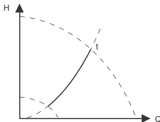
Fig. 28 "Konstant temperatur"
