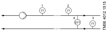
Fig. 40 Overblik over Pt100/1000-sensorens placeringer
