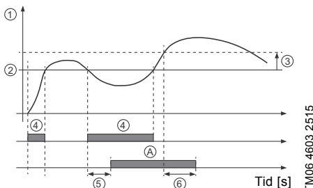
Fig. 51 "Grænse overskredet" (eksempel)
