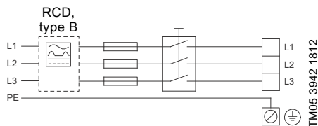
Fig. 6 Eksempel på nettilslutning af en motor med netspændingsafbryder, forsikringer og ekstrabeskyttelse
