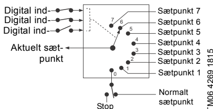
Fig. 50 Principtegning som viser hvordan foruddefinerede sætpunkter fungerer
