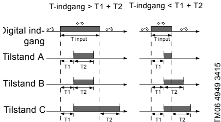
Fig. 43 Analoge indganges varighedsmålingsfunktioner
