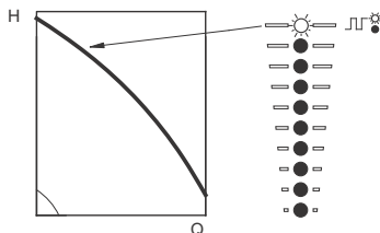
Fig. 18 Drift på maksimumskurven
