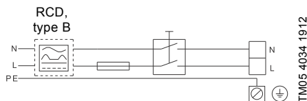
Fig. 4 Eksempel på nettilsluttet motor med netspændingsafbryder, forsikring og ekstrabeskyttelse
