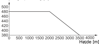
Fig. 13 Forsyningsspænding for 3-faset motor i forhold til højde
