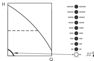
Fig. 19 Drift på minimumskurven
