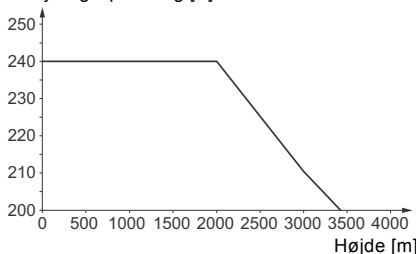
Fig. 14 Forsyningsspænding for 1-faset motor i forhold til højde
