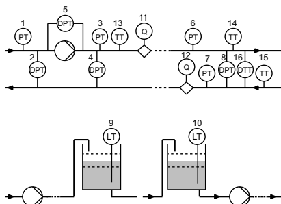
Fig. 39 Overblik over sensorens placeringer
