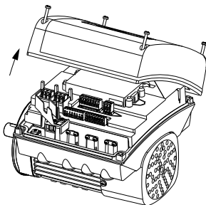
Fig. 65 Sådan afmonteres klemkassedækslet
