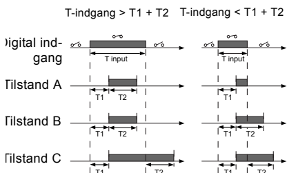
Fig. 41 Analoge indganges varighedsmålingsfunktioner
