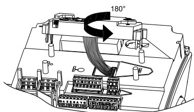
Fig. 67 Sådan drejes plastdækslet
