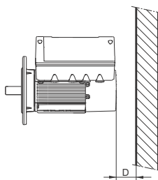
Fig. 1 Minimumsafstand, D, fra motoren til en væg eller andre faste objekter
