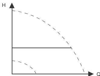
Fig. 26 "Konstanttryk"
