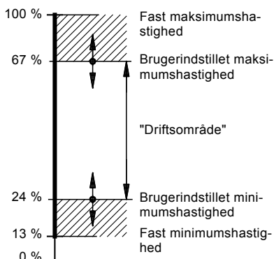
Fig. 44 Eksempel på minimums- og maksimumsindstillinger
