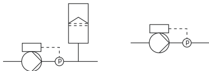
Fig. 27 "Konstanttryk"
