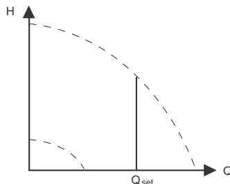
Fig. 34 "Konstant flow"
