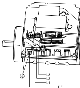
Fig. 7 Nettilslutning, 3-fasede motorer
