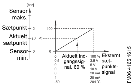
Fig. 45 Eksempel på sætpunktsindflydelse med reguleringssensor
