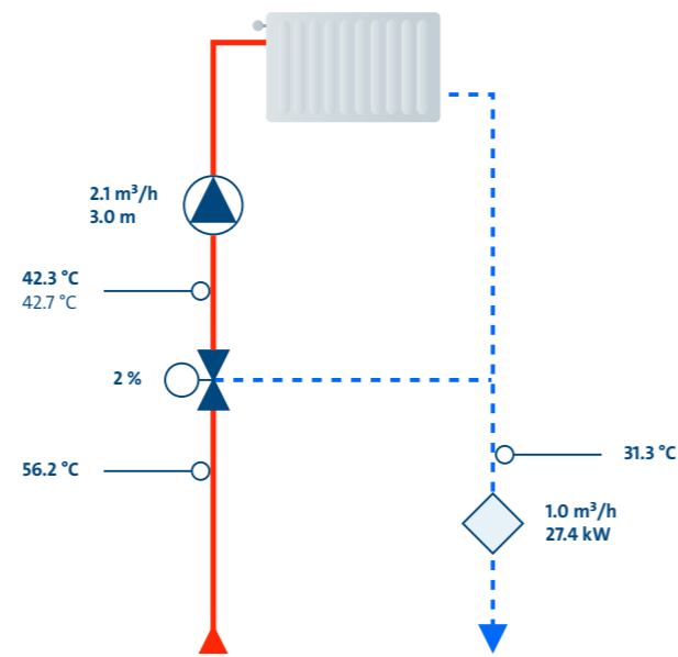
Figur 1: MIXIT DYNAMIC-skema som vist i BuildingConnect.
